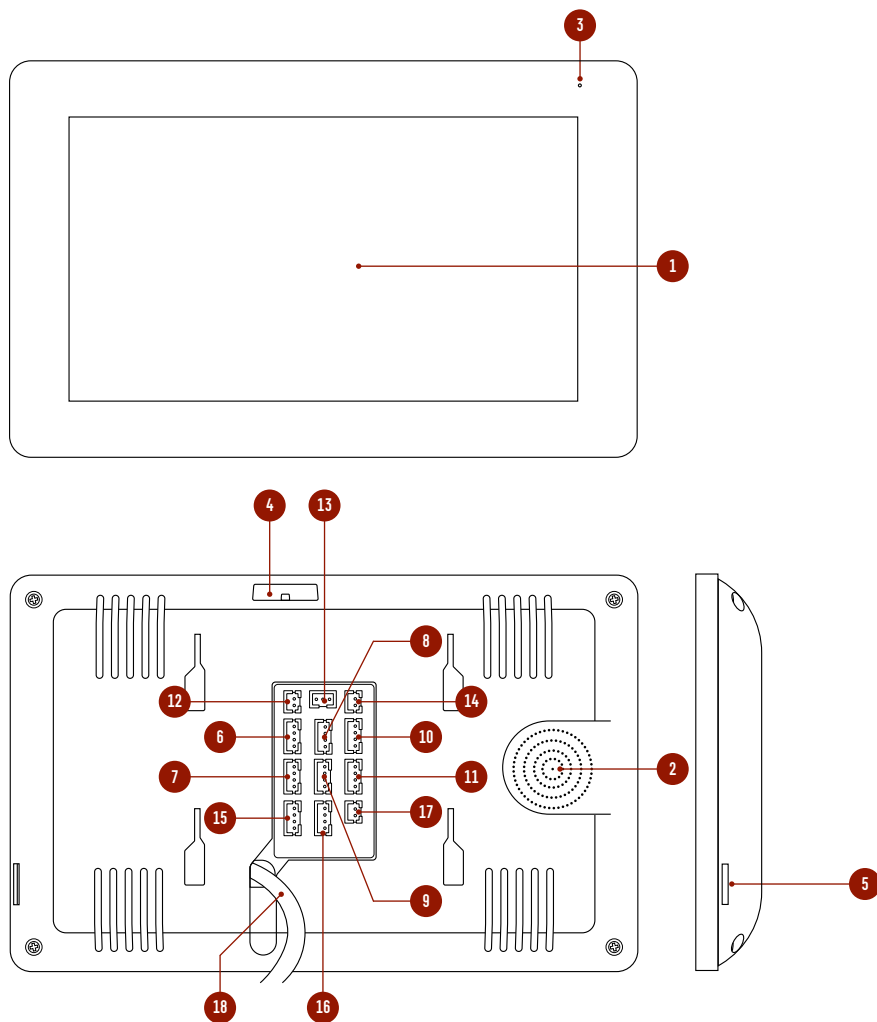
Рис. 4. Описание монитора видеодомофона FREEDOM 7 FHD WIFI
