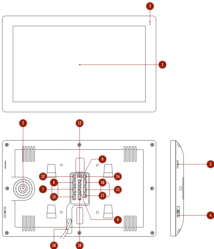
Рис. 5 Описание монитора видеодомофона FREEDOM 10 FHD WIFI
